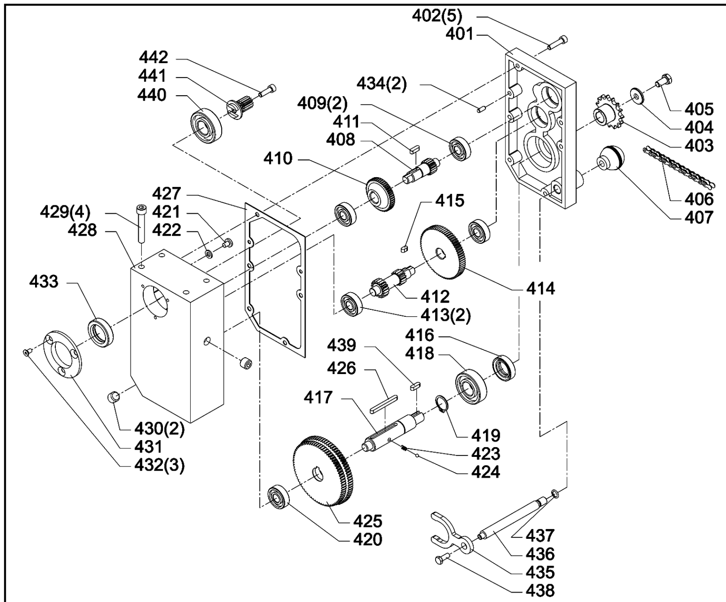
Рис. 3 Детали сборки «Корвет 221М» (Рис.3)
